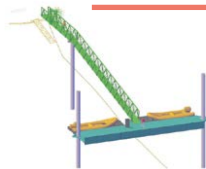
Schéma du nouveau ponton.
